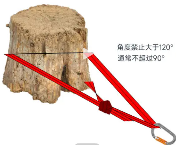
强壮锚单环
